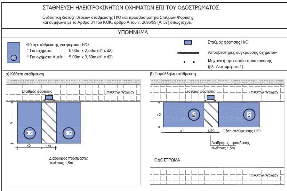
Εικόνα 1.α: Ενδεικτική χωροθέτηση θέσεων στάθμευσης και σταθμών επαναφόρτισης επί οδοστρώματος.
